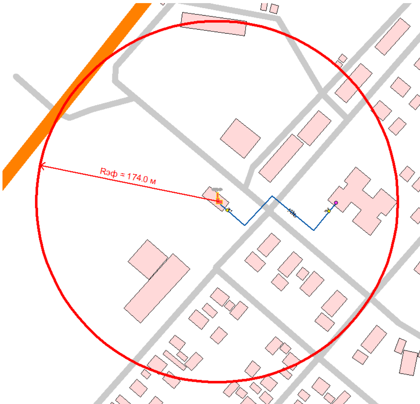
Рис.2 Радиус эффективного действия котельной МУП «Содружество»
